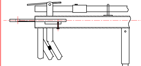
Detalje 1.
